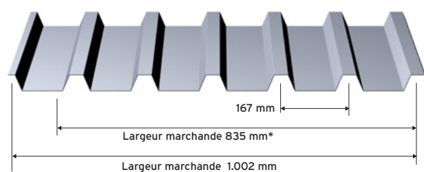
Profil trapézoïdal Aluform 40/167
