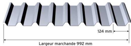
Profil trapézoïdal Aluform 29/124
