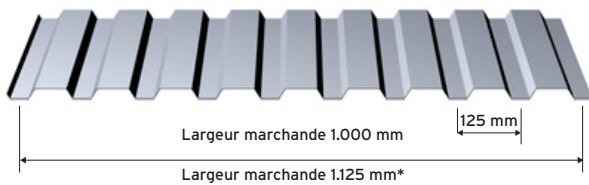
Profil trapézoïdal Aluform 20/125 de préférence comme plafond suspendu
