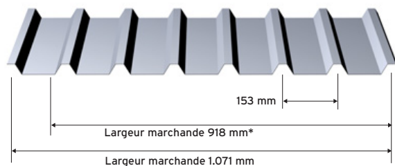
Profil trapézoïdal Aluform 30/153
